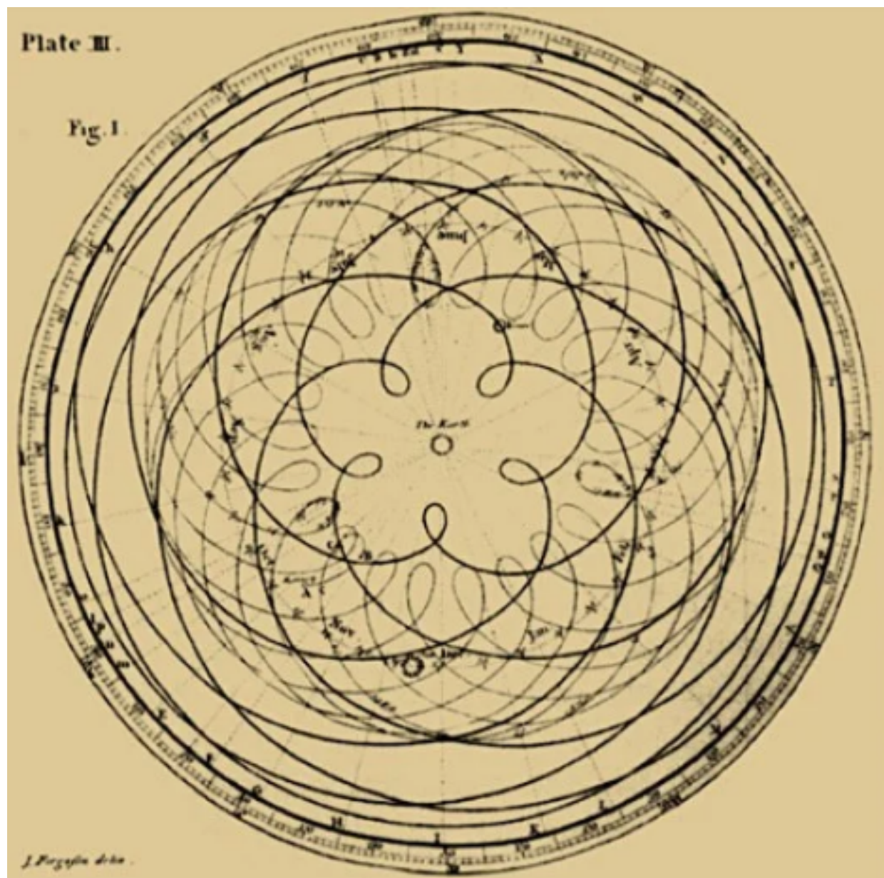
Diagrama del desplazamiento de Venus en el cielo en relación al desplazamiento de la tierra
